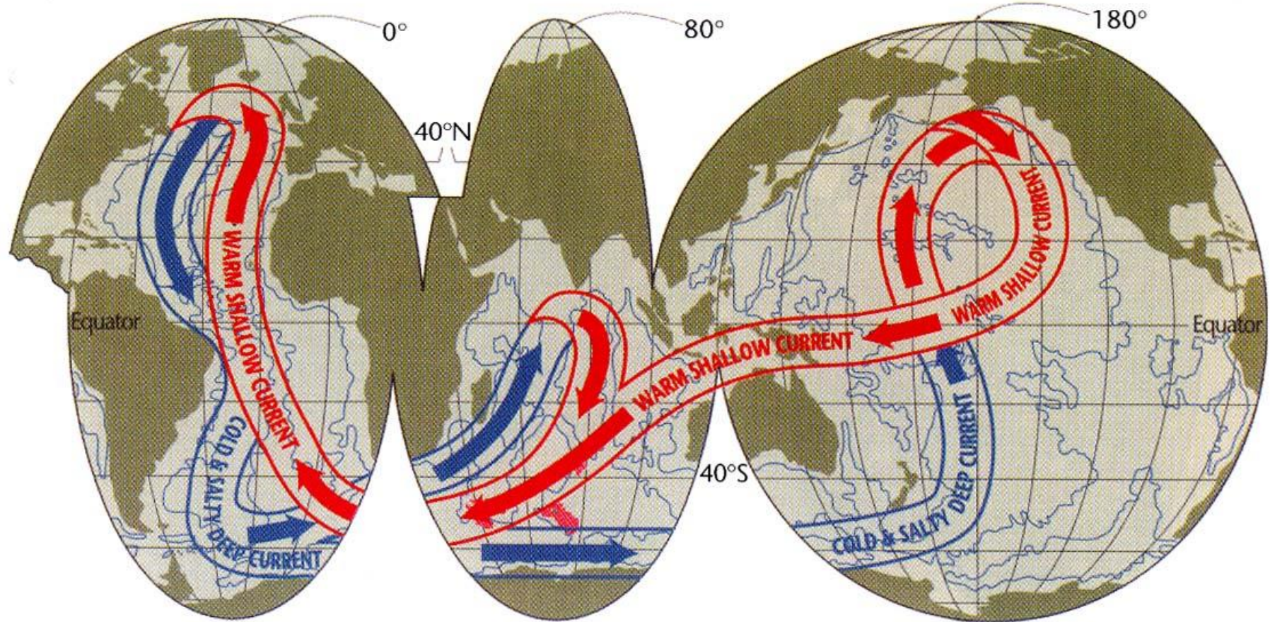
図 5 ブロッカーのコンベアベルト。海洋の深層・表層循環に伴う海水の3次元的な移動を大胆に簡略化して示したもの。Broecker (1987) の原図をもとに Schmitz (1995) が書き直した。 Warm Shallow Current : 高温浅層流, Cold & Salty Deep Current : 低温高塩深層流
