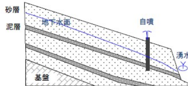
f) 傾斜丘陵地タイプ
