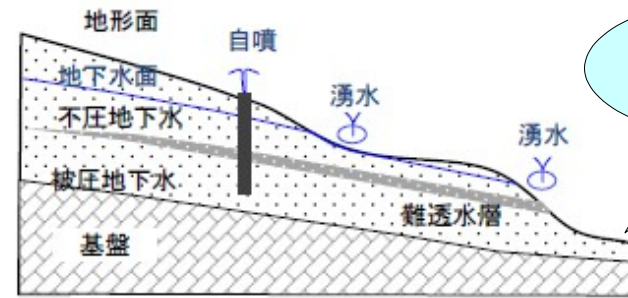
d) 扇端タイプ
