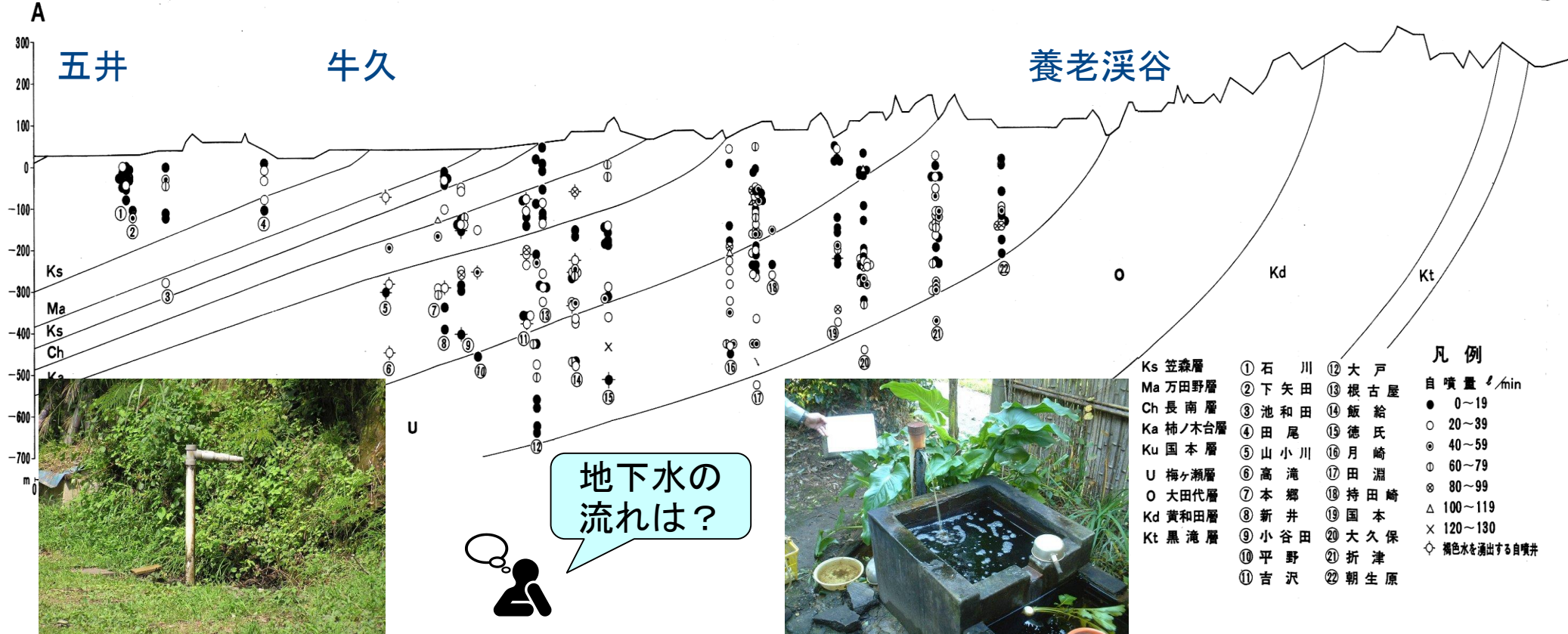
図12-4 地質断面と自噴井の取水深度および自噴量状況図(A-B) (高村原図)
